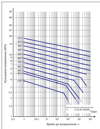
Рис. 1. Эталонные графики длительной прочности PP-R
