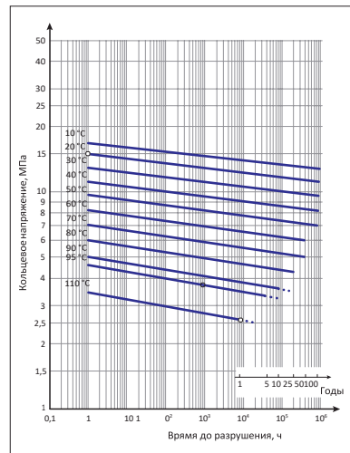
Рис. 2. Эталонные графики длительной прочности PP-RCT
