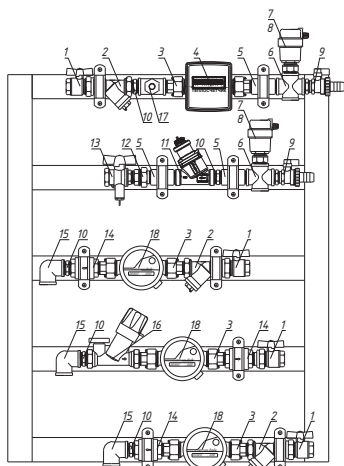
Квартирная станция РОСТЕРМ в горизонтальном исполнении для систем отопления и водоснабжения с рециркуляцией ГВС HWRC-H-LR-15-MD
