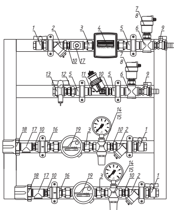
Квартирная станция РОСТЕРМ в горизонтальном исполнении для систем отопления и водоснабжения HW-H-LR-15-MD
