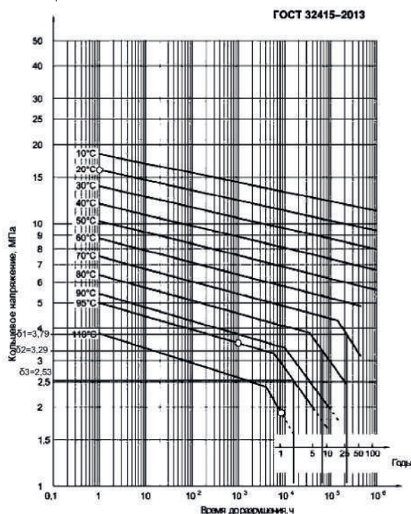
Рисунок В.3 – Стандартные графики длительной прочности PP-R
