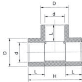
ТРОЙНИК 90°
